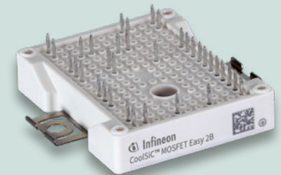
Das CoolSiC™ MOSFET Easy 2B-Modul bietet eine skalierbare Lösung für Fotovoltaik-Wechselrichter und Ladeinfrastruktur für Elektrofahrzeuge.
