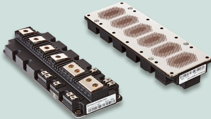
Das PrimePACK™-Modul kommt in Hochleistungs-Wechselrichtern in Windturbinen und Fotovoltaik-Freiflächenanlagen zum Einsatz.
