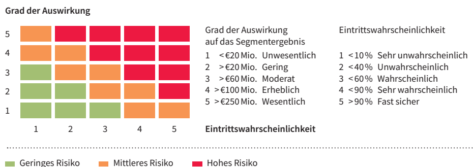
G 78 Risikoklassifizierungsmatrix
